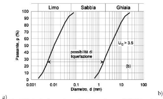
Fig. 7.11.1 – Fusì granulometrici di terreni suscettibili di liquefazione
